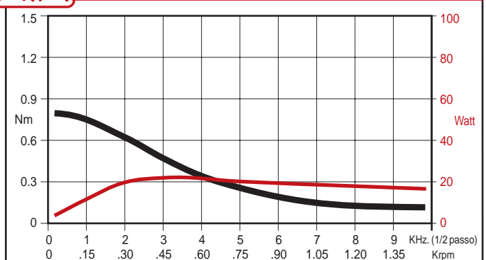
SANYO 103 714 0150 collegamento unipolare 24 Volt, 1,8 Amp.
