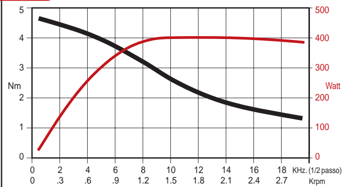
SANYO 103 845 6741 - coll. bipolare parallelo Azionamento RTA GMD04
