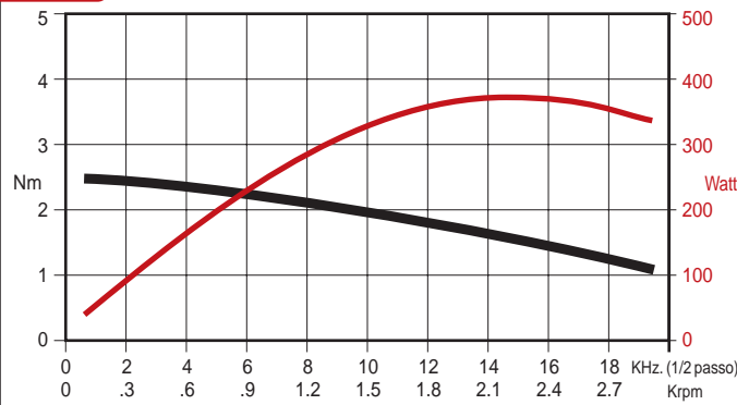
SANYO 103 H8221 6241 - coll. bipolare Azionamento RTA GMD04
