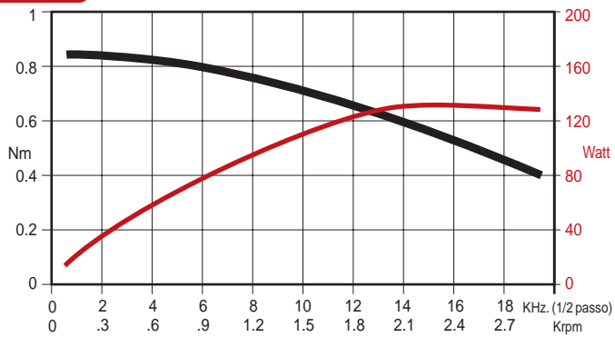
SANYO 103 H7123 1740 - coll. bipolare Azionamento RTA GMD02
