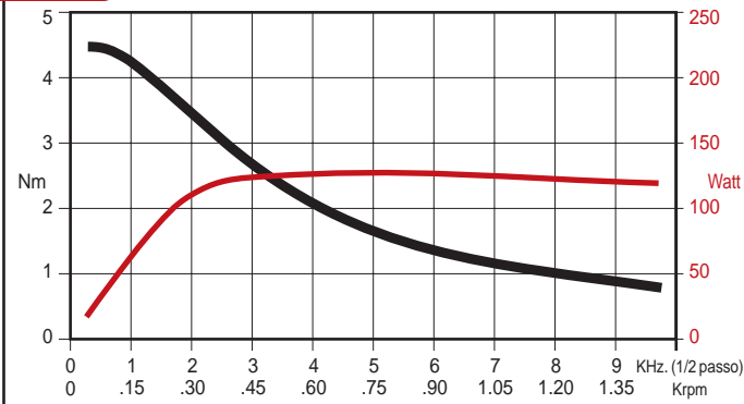
SANYO 103 845 6741 - coll. bipolare serie Azionamento RTA GMD02
