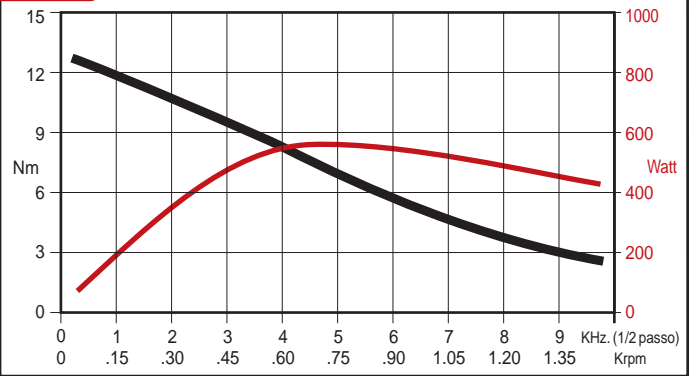
SANYO 103 8960 6551 - coll. bipolare parallelo Azionamento RTA GMD03
