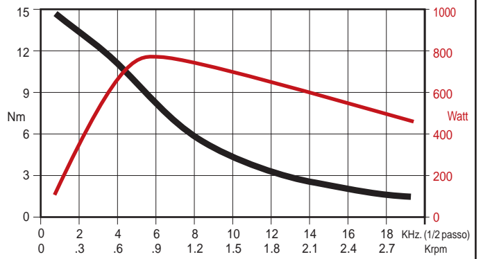
SANYO 103 8960 6551 - coll. bipolare parallelo Azionamento RTA GMD04
