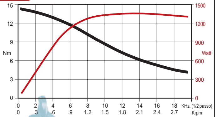
SANYO 103 8960 6551 - coll. bipolare parallelo Azionamento RTA BCW02
