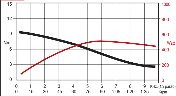
SANYO 103 8932 6451 - coll. bipolare parallelo Azionamento RTA GMD03
