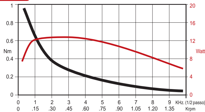
SANYO 103 H7126 0140 collegamento unipolare 24 Volt, 1 Amp.
