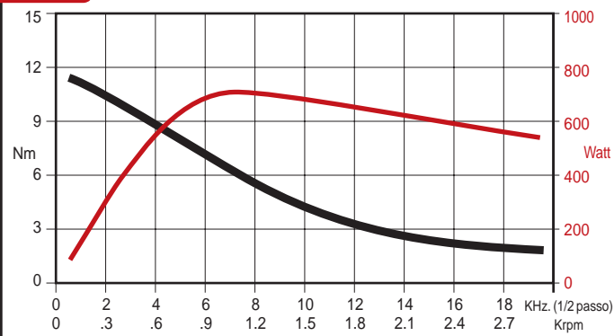
SANYO 103 8932 6451 - coll. bipolare parallelo Azionamento RTA GMD04
