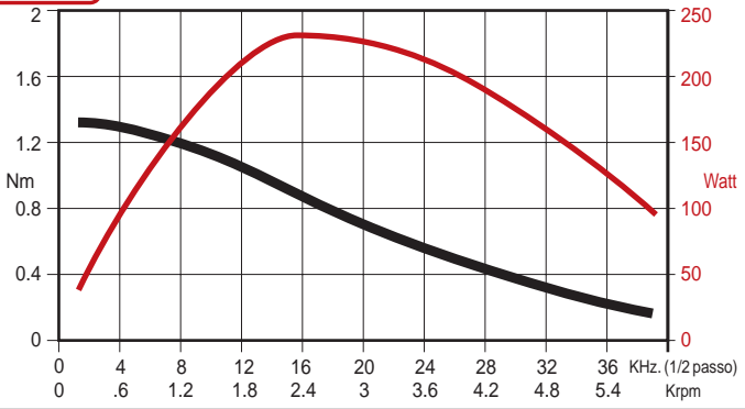
SANYO 103 H8221 6241 - coll. bipolare Azionamento RTA GMD02
