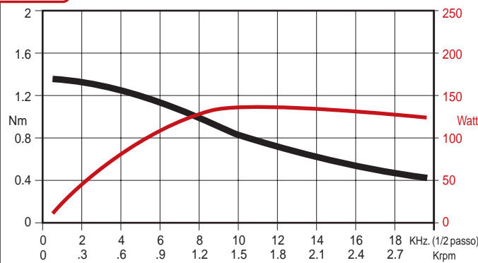
SANYO 103 H7126 1740 - coll. bipolare Azionamento RTA GMD02
