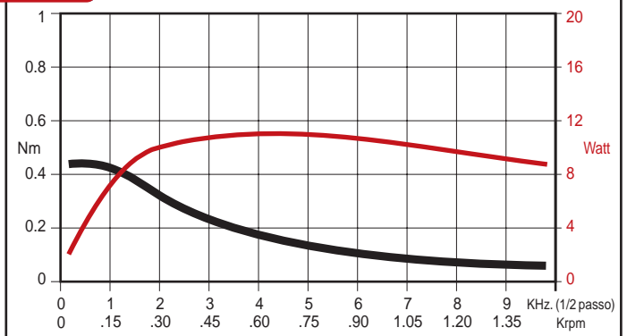
SANYO 103 770 6 collegamento unipolare 24 Volt, 1 Amp.
