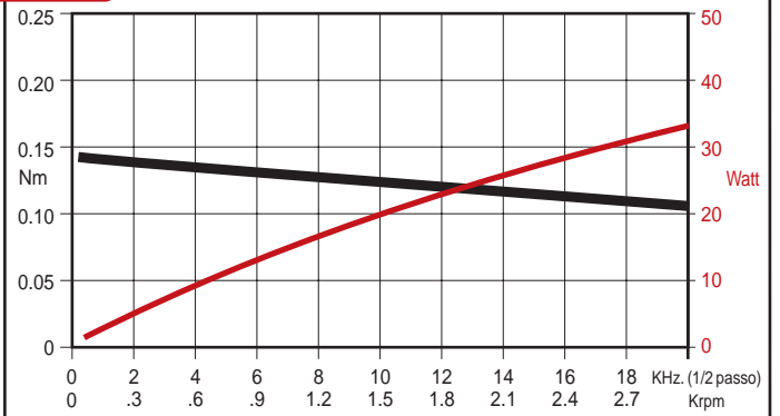
SANYO 103 547 52500 - coll. bipolare parallelo Azionamento RTA NDC04
